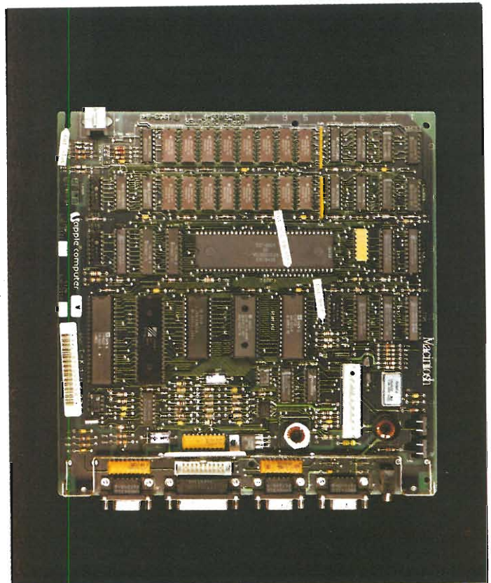
Qui sono indicate le piste da tagliare sulla faccia superiore della scheda principale del Mac.
