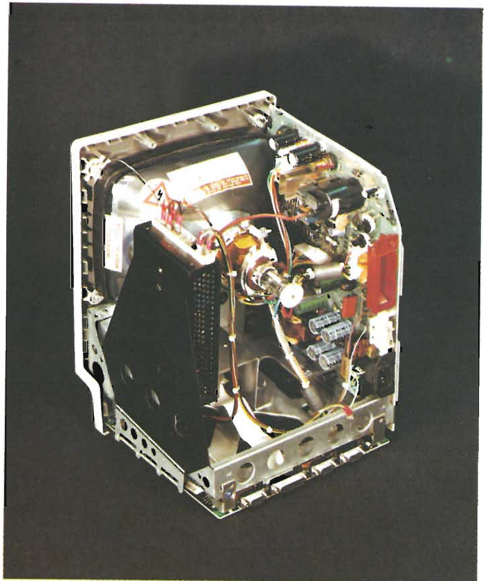
Il nuovo alimentatore installato all'interno del Mac.
