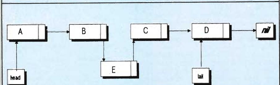
Fig. 3. Inserzione di un elemento in una lista a puntatori.
