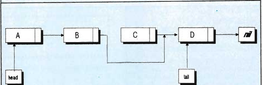
Fig. 1. Una tipica lista lineare a puntatori.
