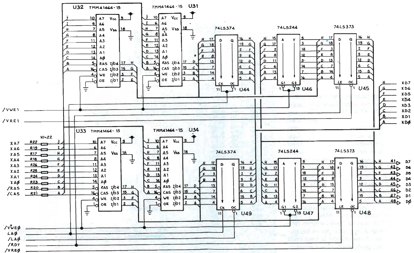
Fig. 12. Banco della memoria video.
